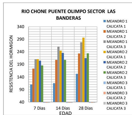
Figura 10. Resistencias del diseño de Hormigón de 240 kg/cm 2 propuesto con agregado grueso de la cantera La Chicha con el Río Chone puente Olimpo sector Las Banderas.
