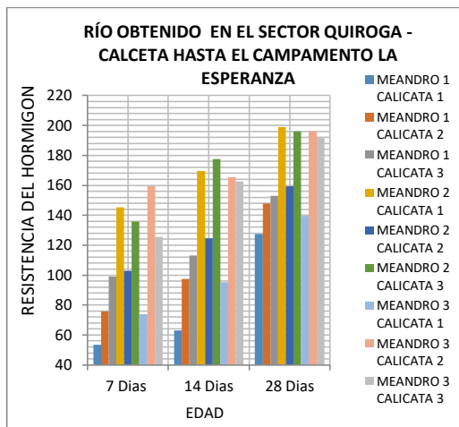
Figura 6. Resistencias del diseño de Hormigón de 240 kg/cm 2 propuesto con agregado grueso de la cantera Megarock y con agregado fino del río obtenida en el sector Quiroga-Calceta hasta el campamento la esperanza.
