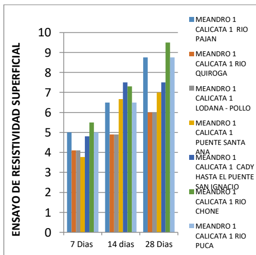
Figura 12. Resultados de ensayos de Resistividad superficial proveniente de los Ríos de la Provincia de Manabí
