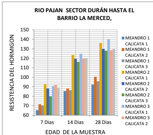
Figura 5. Resistencias del diseño de Hormigón de 240 kg/cm 2 propuesto con agregado grueso de la cantera San Agustín y con agregado fino del río Paján sector Durán hasta el barrio la Merced.
