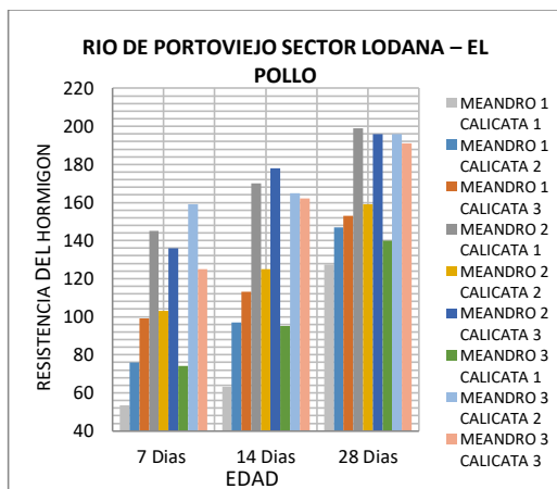
Figura 7. Resistencias del diseño de Hormigón de 240 kg/cm 2 propuesto con agregado grueso de la cantera San Agustín y con agregado fino del río Portoviejo Sector Lodana - El Pollo.
