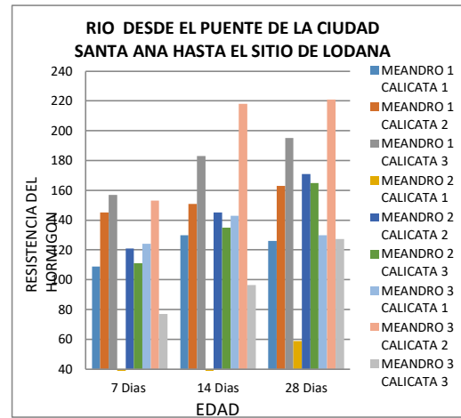
Figura 8. Resistencias del diseño de Hormigón de 240 kg/cm 2 propuesto con agregado grueso de la cantera Grano de Oro y con agregado fino del río desde el Puente de la ciudad Santa Ana hasta Lodana.
