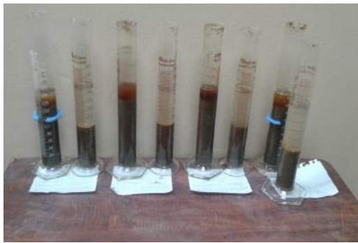
Figura 3. Ensayo de impureza organica.
