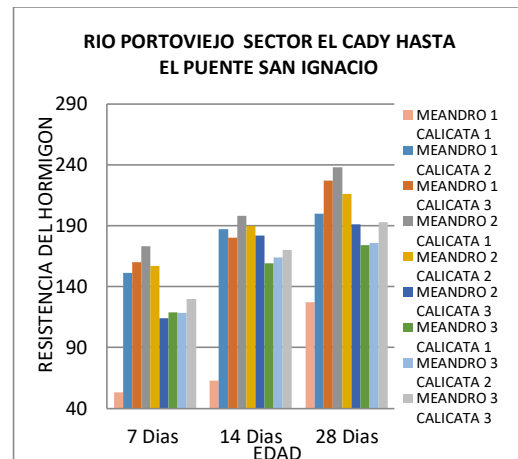
Figura 9. Resistencias del diseño de Hormigón de 240 kg/cm 2 propuestos con agregado grueso de la cantera Megarock con agregado fino del Río Portoviejo sector el Cady hasta el Puente San Ignacio.
