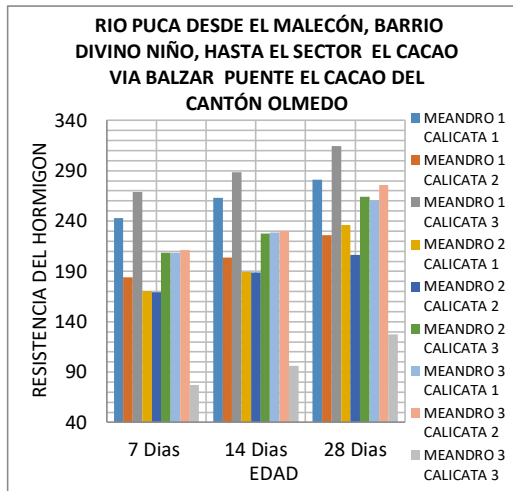
Figura 11. Resistencias del diseño de Hormigón de 240 kg/cm 2 propuesto con agregado grueso de la cantera San José Sector Picoaza con agregado fino del Rio Puca desde el malecón, Barrio Divino Niño, hasta el sector El Cacao Vía Balzar Cantón Olmedo.
