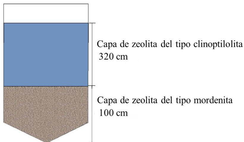
Figura 3. Dimensiones del filtro de zeolita
